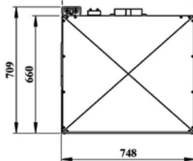
نمای بالا
