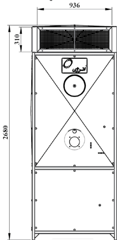
نمای روبرو
